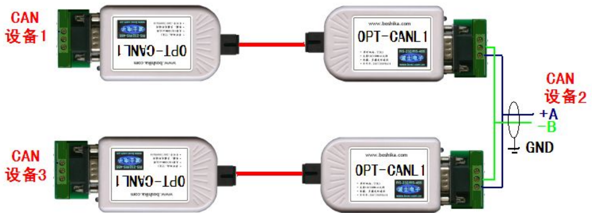
图 3 单纤多机通信
