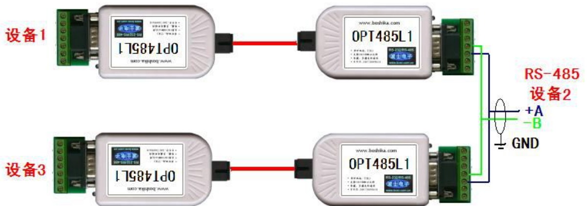
图 3 单纤多机通信
