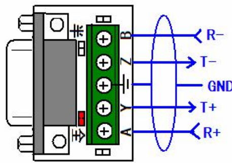
RS-422 全双工
