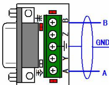
RS-485 半双工
